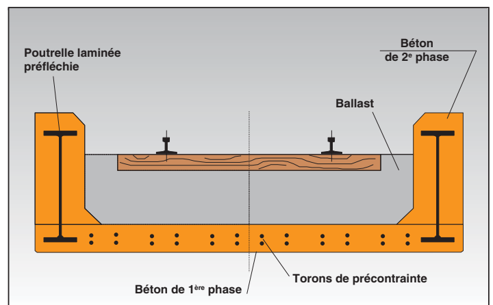
Coupe transversale d'un tablier à poutres latérales préfléchies (schéma de principe). - Ce système ingénieux de tablier entièrement préfabriqué associant préflexion, précontrainte et mixité a été développé par la Société Nationale des Chemins de Fer Belges. (SNCB NMBS)
