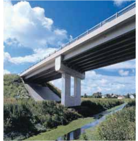
Reconstruction du pont sur la Nahe à Bad Münster am Stein, Allemagne. – Un tablier mixte a été construit sur les piles existantes pour cet ouvrage situé dans une réserve naturelle.
