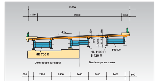
Exemple d'une coupe transversale d'un tablier à 6 poutres maîtresses (contournement de la ville de Luxembourg).
